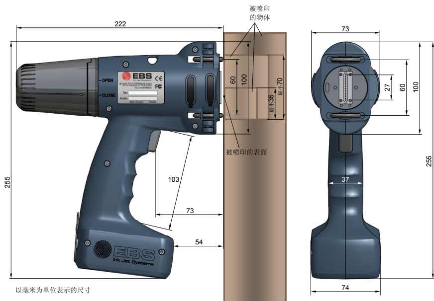
工作状态下喷码机尺寸（侧视及前视图）
